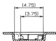
SECT.E-E
