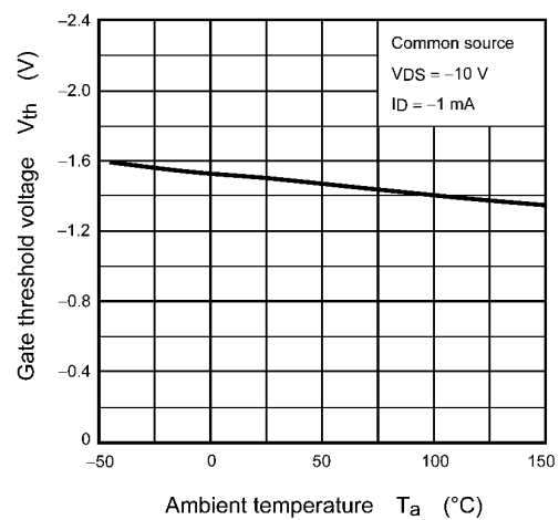
Fig. 8.6 V_{th} - T_a
