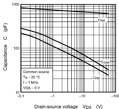
Fig. 8.8 C - V_{DS}
