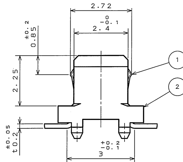
( SCALE 10 : 1 )
