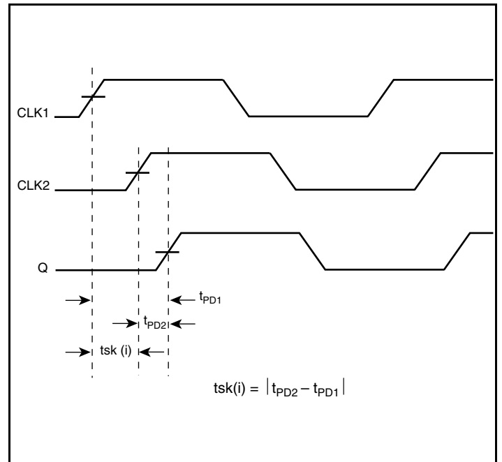
Input Skew
