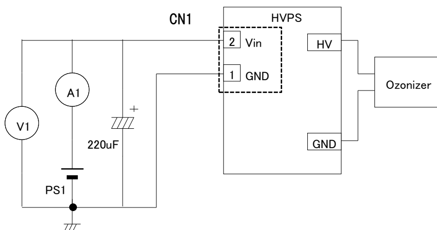
《 図 2 》 推奨回路
