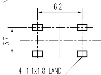
P.C.B 安装位置尺寸 P.C.B LAND DIMENSION
