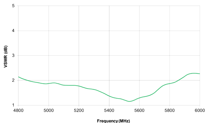
5 GHz VSWR
