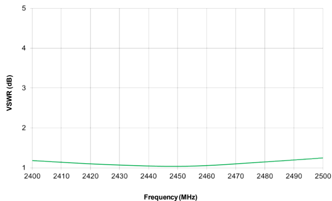
2.4 GHz VSWR
