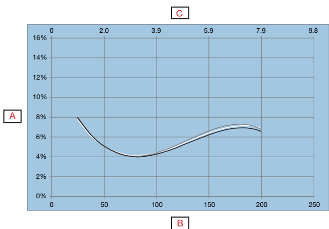
Fig. 6 PD30CTBR20BPxxIO
