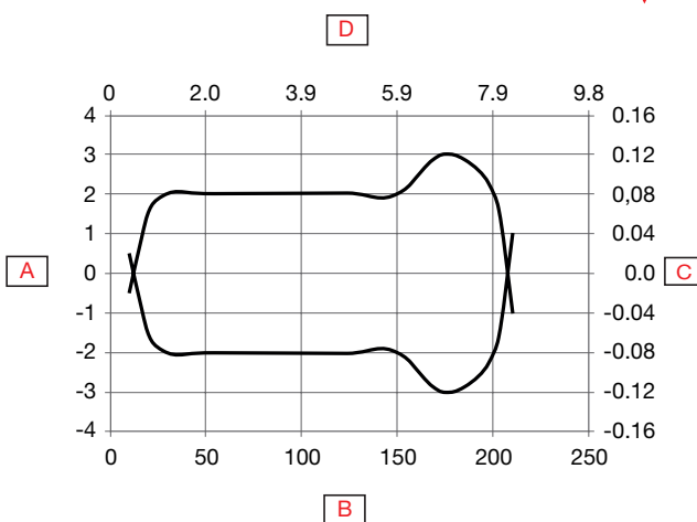
Fig. 5 PD30CTBI20BPxxIO
