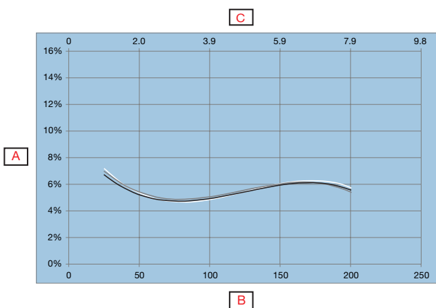
Fig. 7 PD30CTBI20BPxxIO
