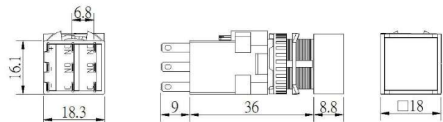
M6L-B (Square)
