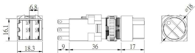
M6S-A (Round)
