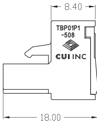
2 Pole Module
