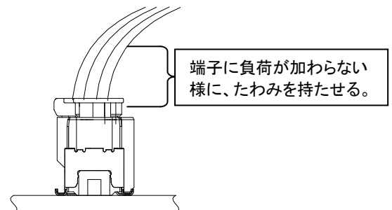
Fig.11 電線にたわみを持たせた状態
