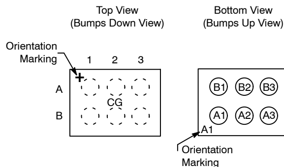
CM1418 WLCSP6 Package
