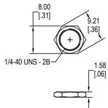
1/4 - 40 Hex Nut
