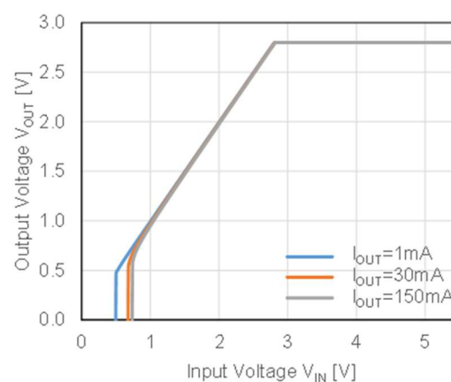
RP123x28xx
