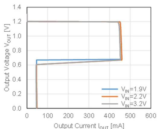
RP123x12xx
