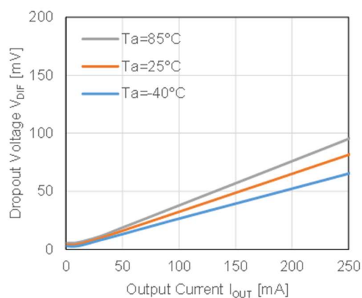
RP123Z28xx
