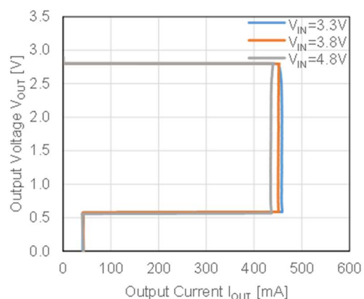
RP123x28xx
