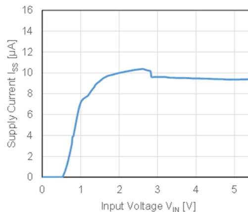
RP123x28xx
