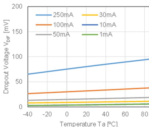
RP123Z28xx
