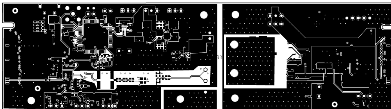
Figure 6-8. Bottom Layer
