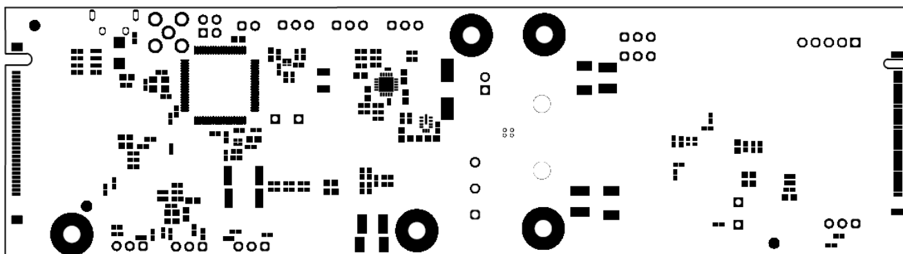
Figure 6-9. Bottom Layer Mask
