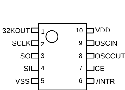
R2043T(TSSOP10G)
