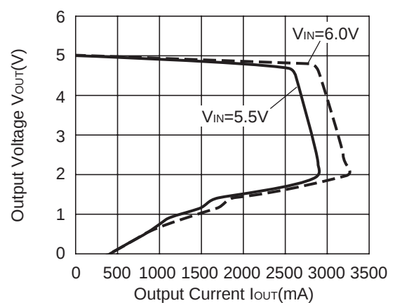
R1171J501x
