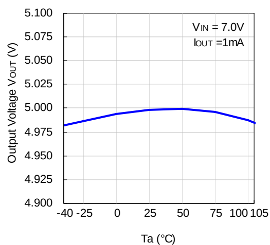
R1511x050B
