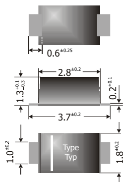
Dimensions - Maße [mm]
