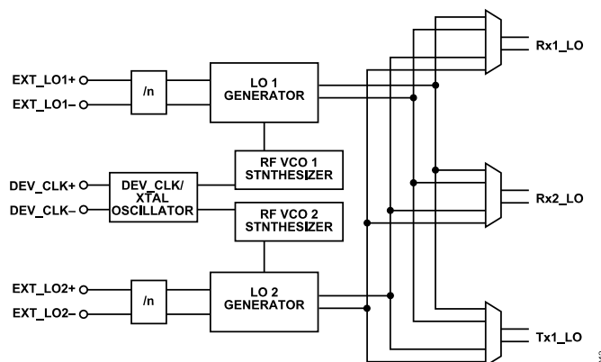
Figure 300. RF LO
