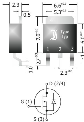
Dimensions - Maße [mm]
