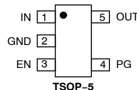
TSOP-5
