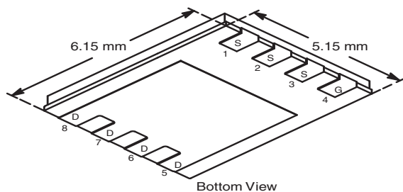
PowerPAK ® SO-8
