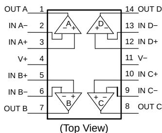
SOIC-14
